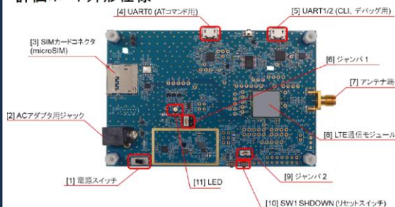
評価ボード外形仕様
